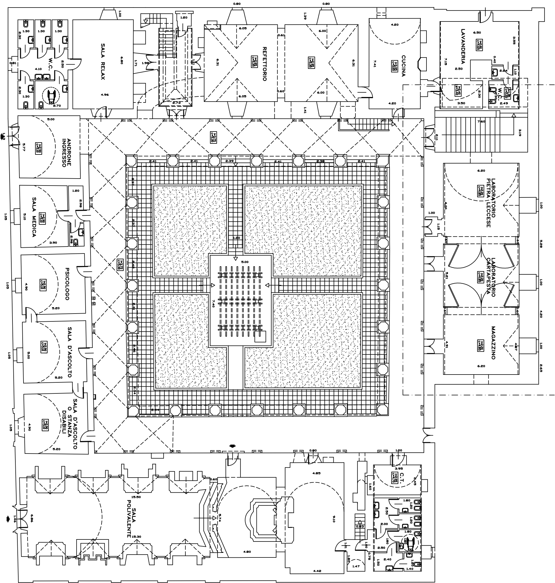
Pianta PIANO interrato
