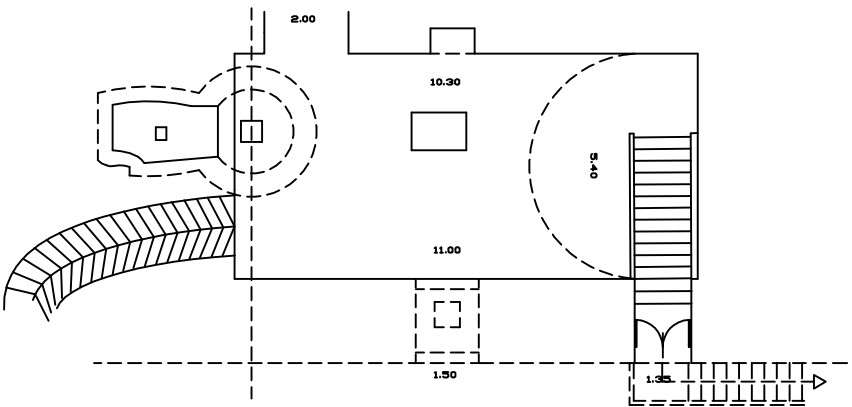
Pianta PIANO interrato
