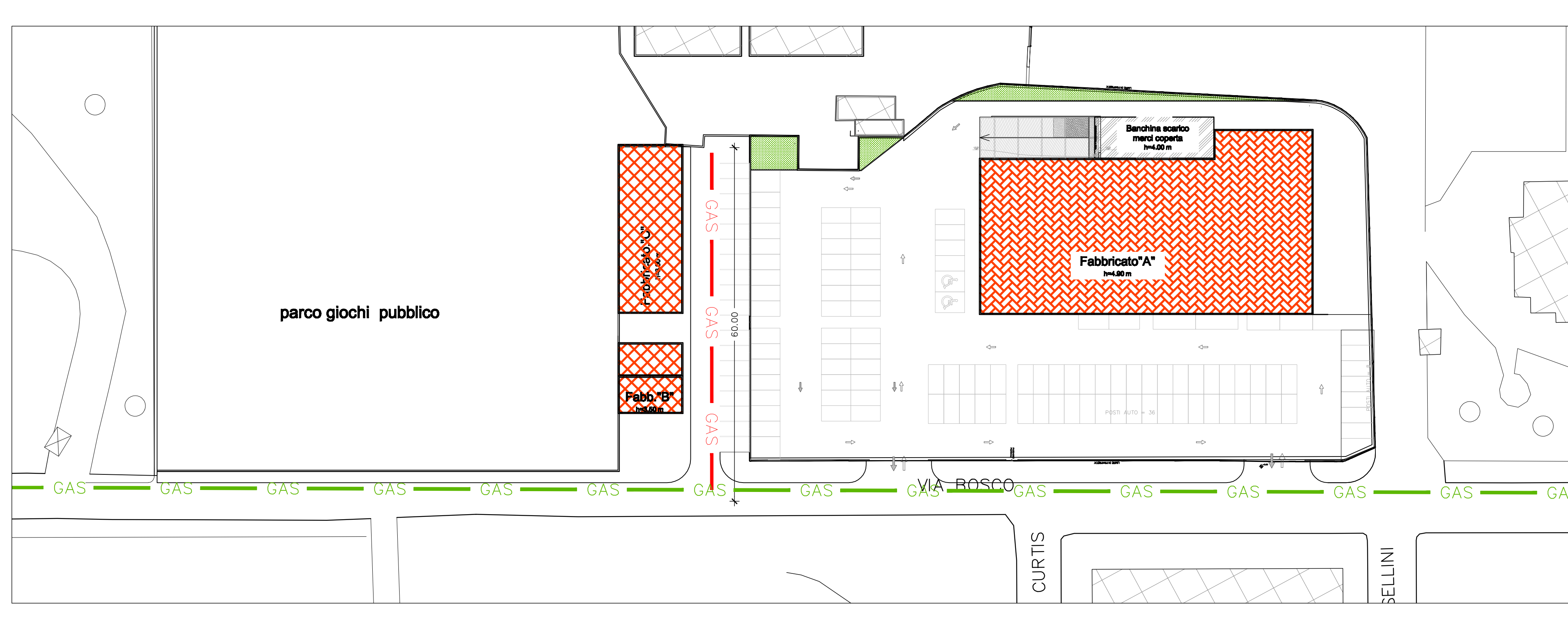
SCHEMA OPERE DI URBANIZZAZIONE PRIMARIA VIA BOSCO RETE GAS - scala 1:500
